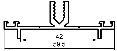
No : 3689 Düşey-Yatay Alt Profili 0,530 kg/m
