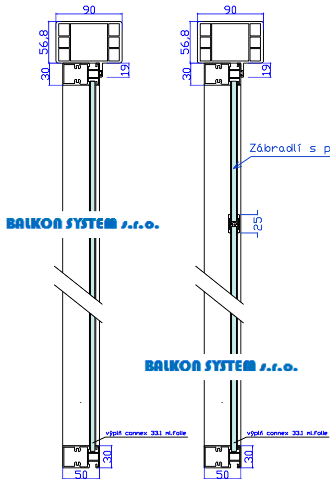
Zábradlí montované z fixního profilu
