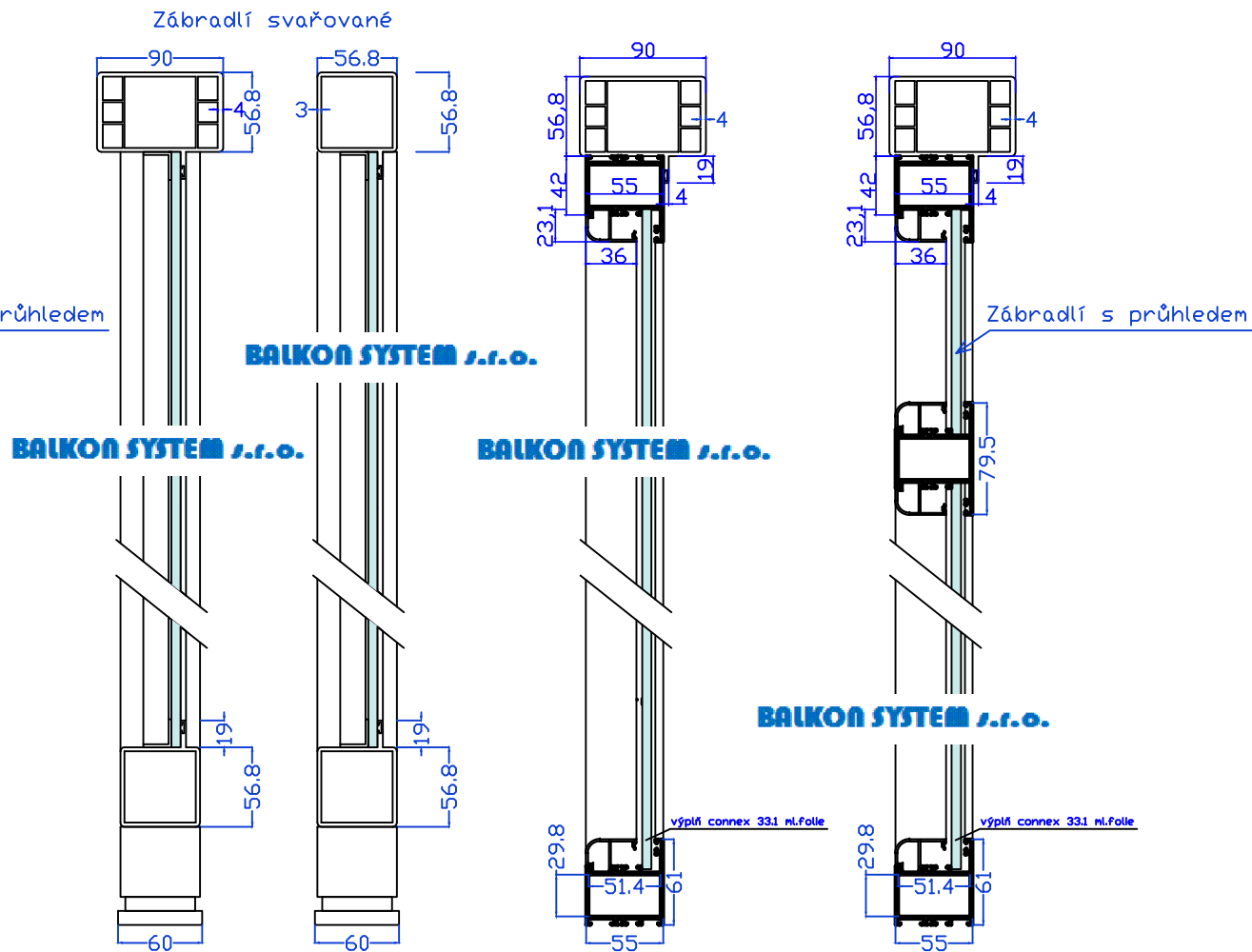
Zábradlí montované z profilů
